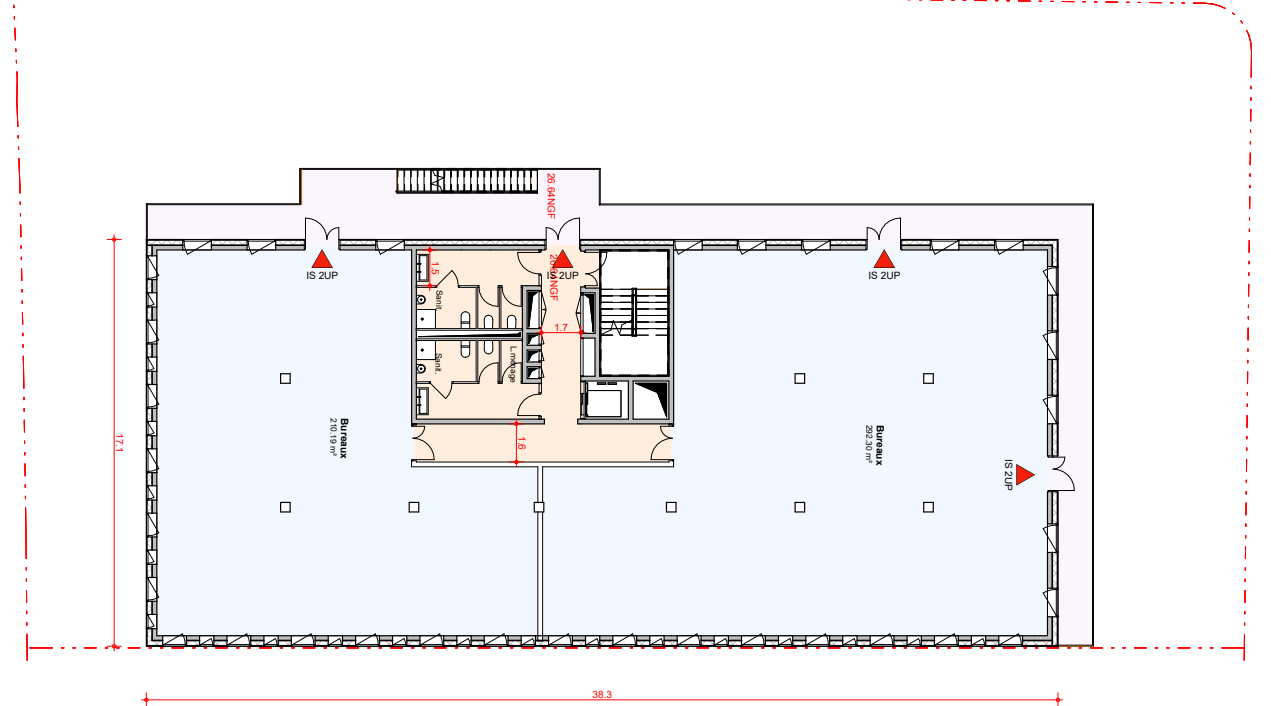
Plan étage courant SUBL 630 m 2
