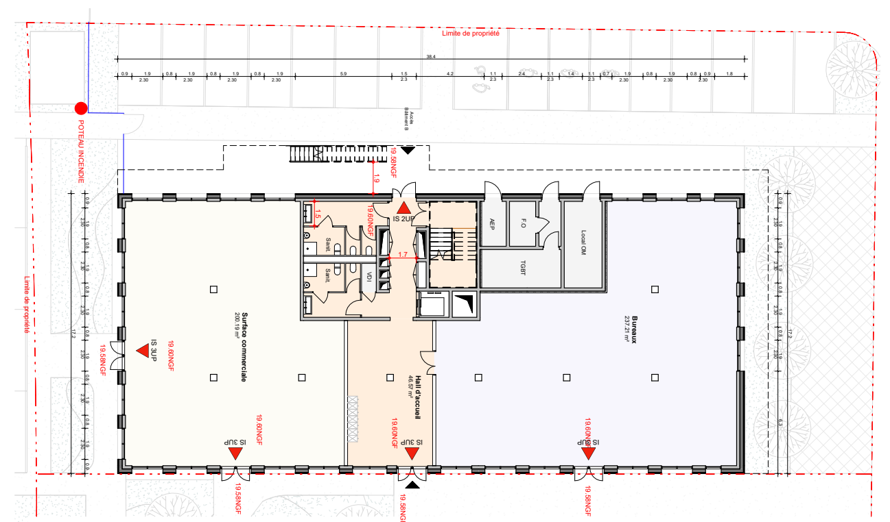
Plan RDC
